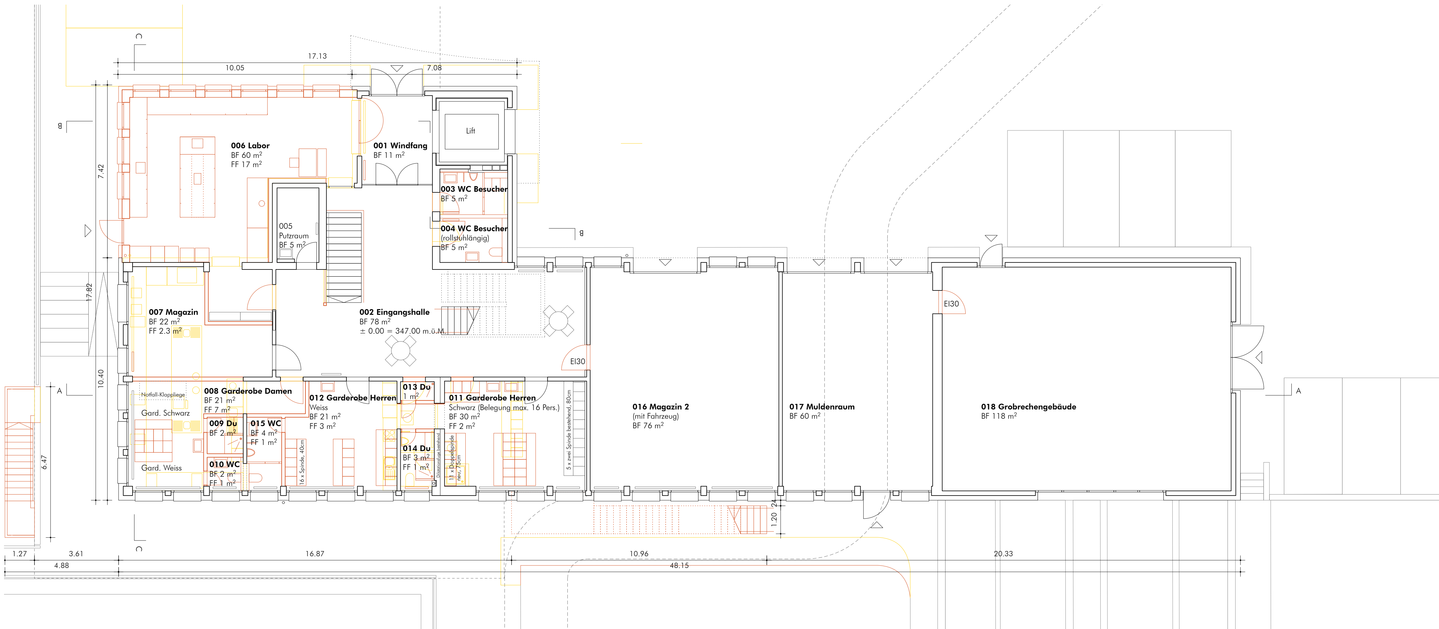
Erdgeschoss
