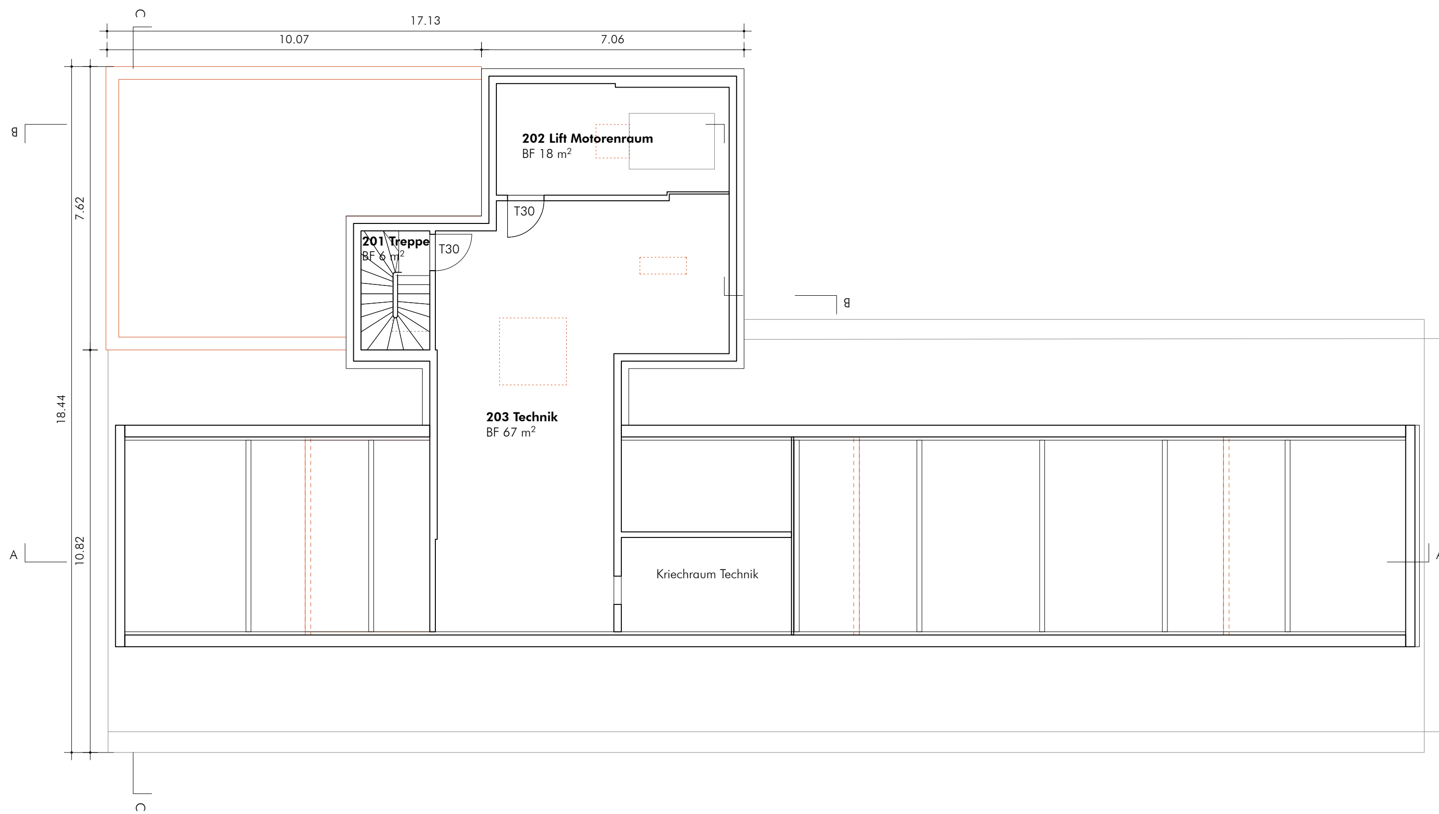
2. Obergeschoss (Technikgeschoss)
