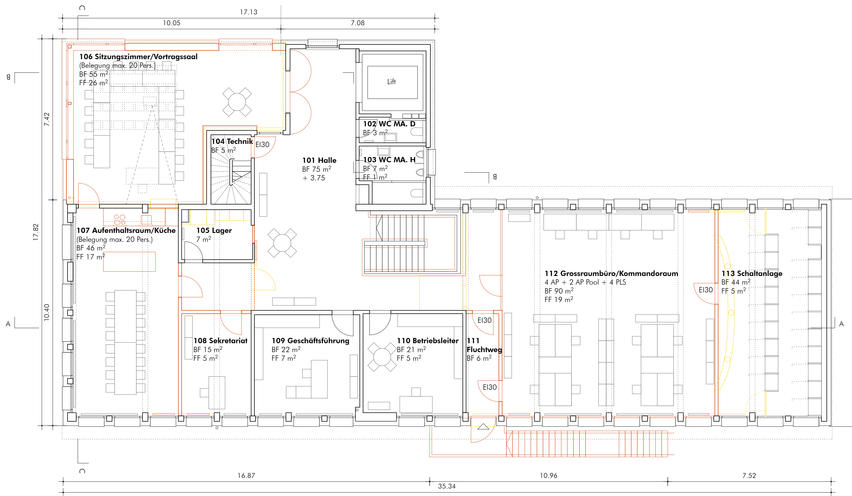
1. Obergeschoss
