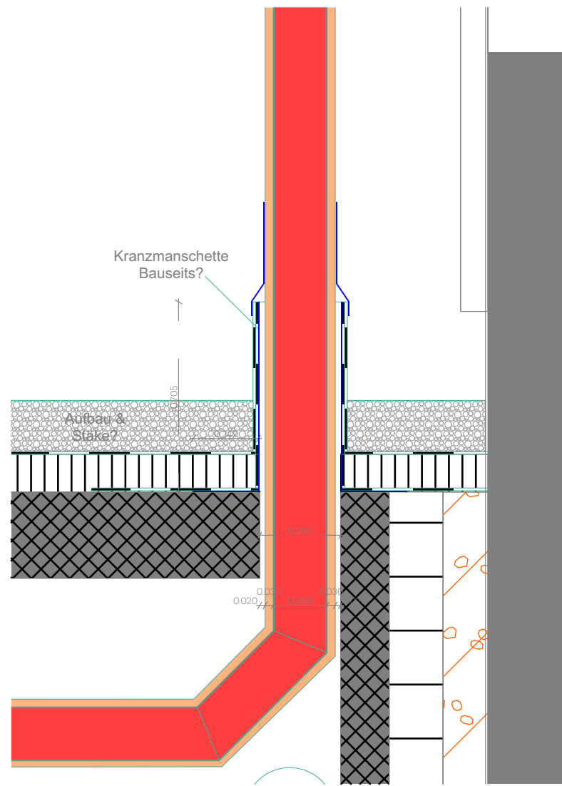
S-02 Gebäudeschnitt 1:20
