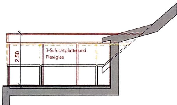
Schnitt 1:100
