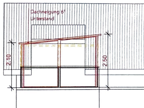
Ansicht 1:100
