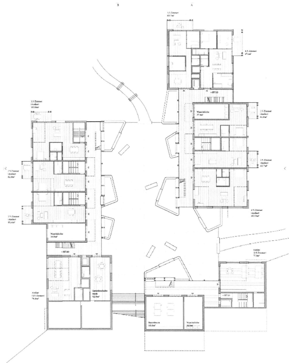
Abbildung 12: Grundriss Platzgeschoss, Cluster West, Siegerprojekt "Kandalama" (Quelle: Projektverfasser)
