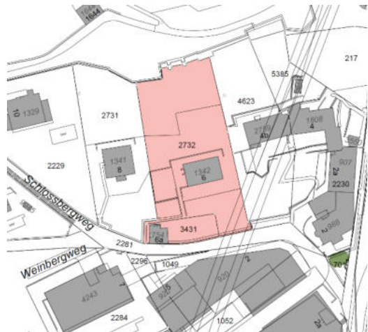
Situation, Maßstab ca. 1:1'500
