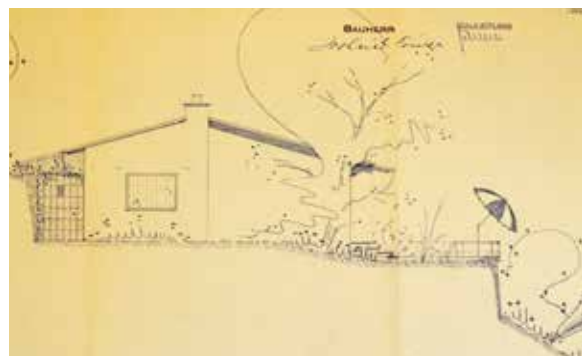
Baueingabeplan 1950
