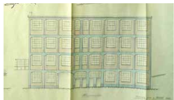
Baueingabeplan 1909
