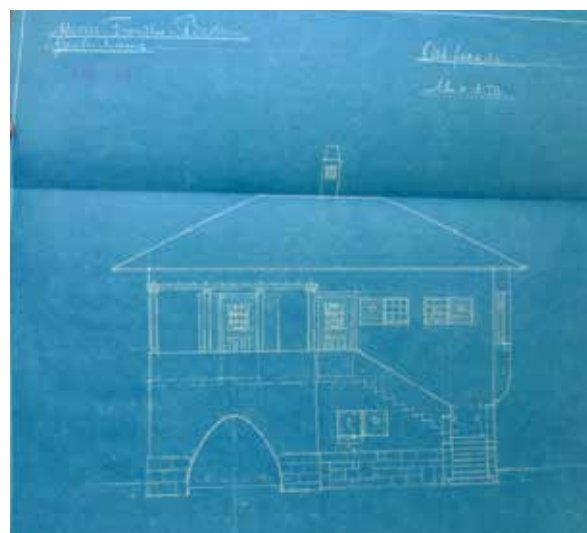
Baueingabepläne für das Gartenhaus
