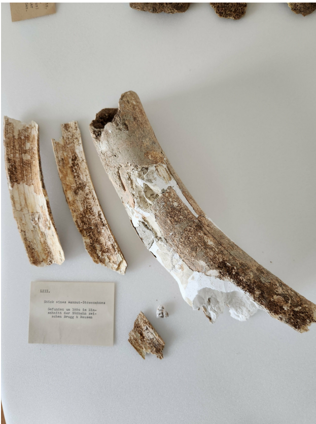
Bildlegende: Stück eines Mammut-Stosszahnes, gefunden um 1890 im Einschnitt der Südbahn zwischen Brugg und Hausen
